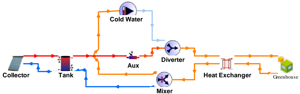
Fig. 5: Diagrama en TRNSYS 17 del sistema de climatización.
