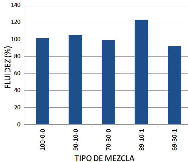
Figura 8. Fluidez de morteros
