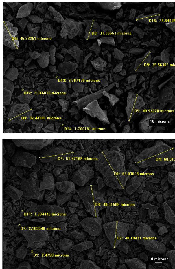
Figura 6. SEM Ceniza de Cascarrilla de arroz (sup) y Cemento Portland Ordinario (inf) (X500)
