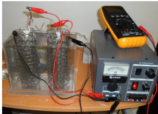
Figura 4. Arreglo experimental de CA con corriente impresa
