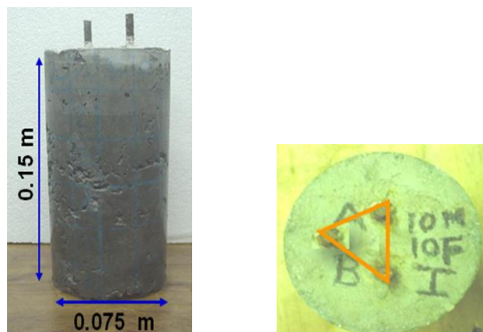
Figura 1. Esquema del espécimen empleado
