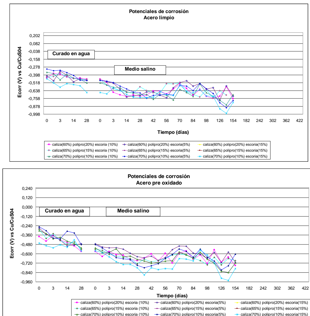
Figura 5. Potenciales de corrosión de los especímenes con agregado calizo - polipropileno -escoria (10, 5, 15%).
