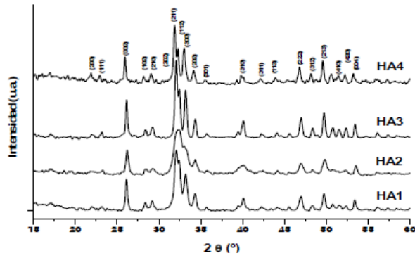
Figura 1. Difractogramas de rayos X de las diferentes muestras sintetizadas.
