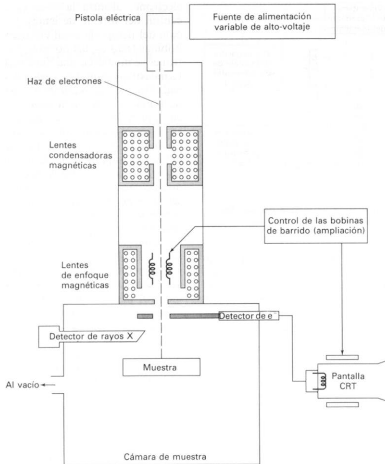
Figura 2.13. Esquema de microscopio electrónico de barrido (SEM).
