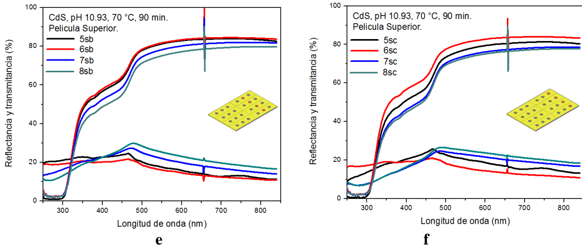
Figura 3.3. Gráficas de T&R de películas superiores de la serie X a. 1a, 2a, 3a y 4a. b. 1b, 2b, 3b y 4b. c. 1c, 2c, 3c y 4c. d. 5a, 6a, 7a y 8a. e. 5b, 6b, 7b y 8b. f. 5c, 6c, 7c y 8c.
