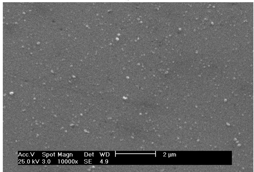
Figura 3.19. Imágenes de SEM con aumentos de 10000X de la película SUPERIOR 3b de la serie: a) X (pH 10.93), b) Y (pH 11.58) y c) Z (pH 12.18)
