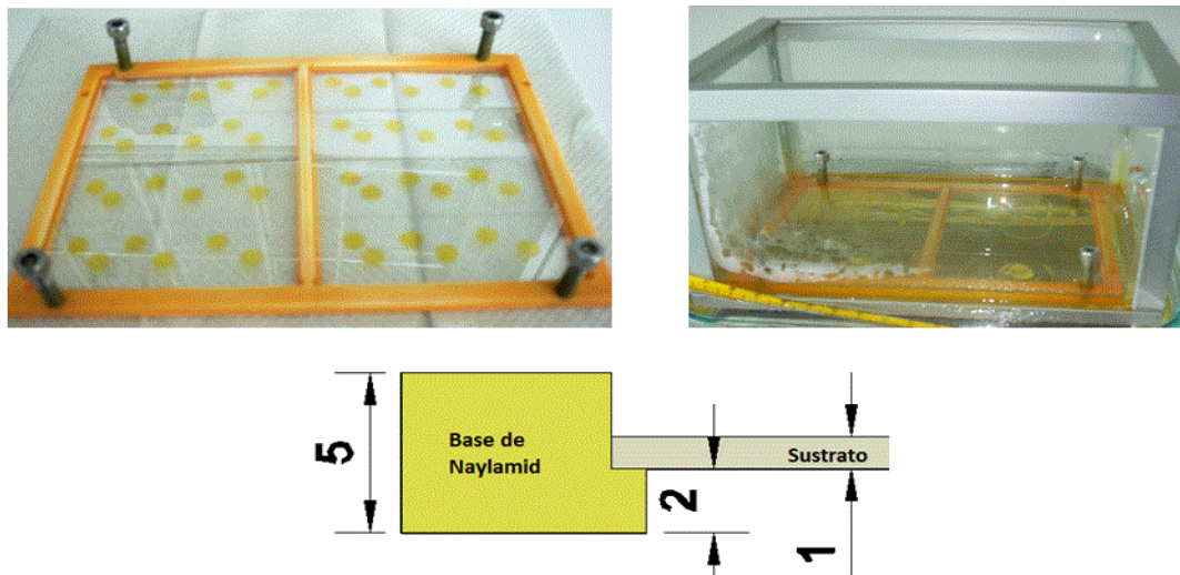
Figura 2.1. Izq. portaobjetos con cinta kapton sobre la base de nylamid. Der. Recipientes utilizados para el baño químico. Inf. Dimensiones (en mm) de la base de Naylamid.
