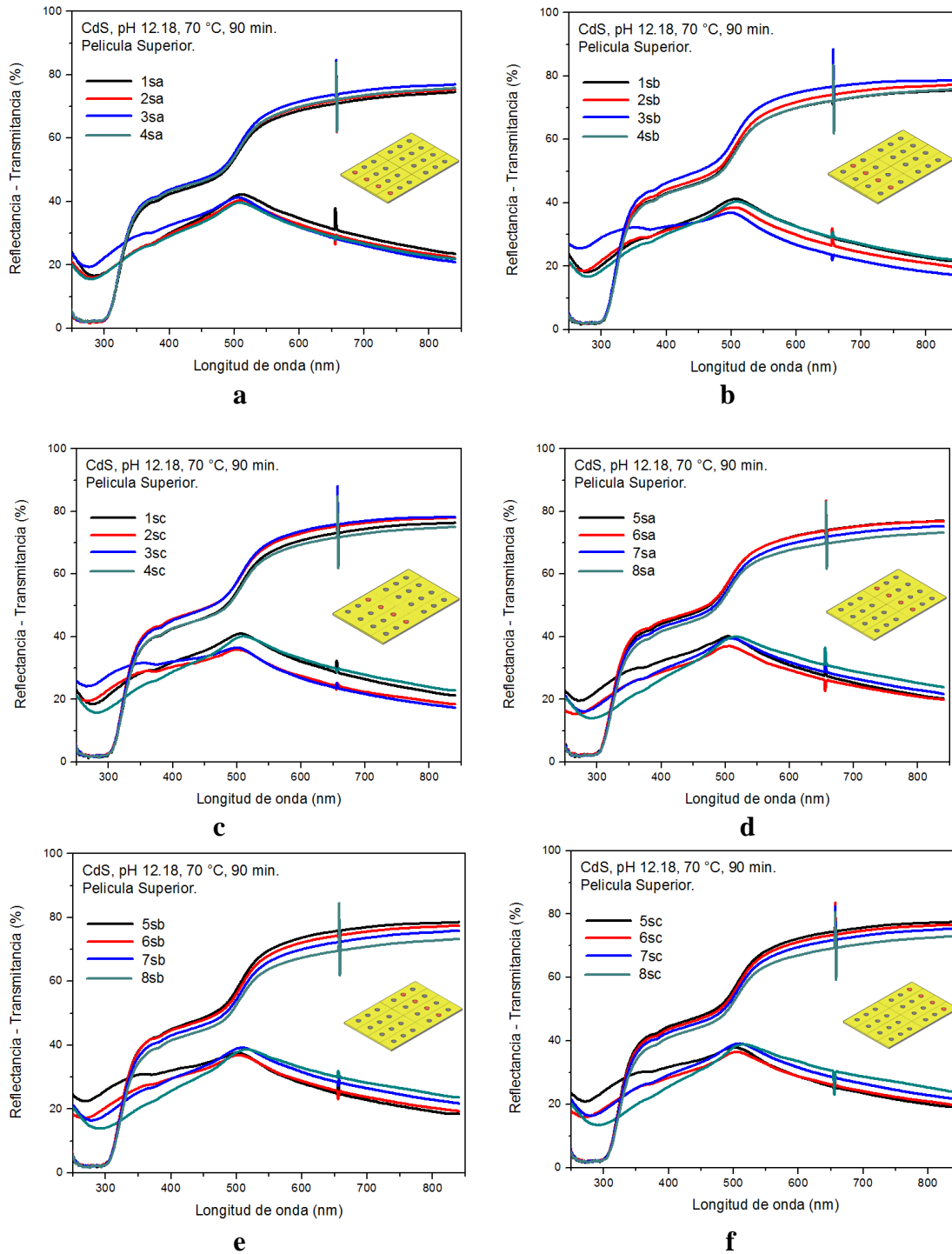
Figura 3.7. Gráficas de T&R de películas superiores de la serie Z a. 1a, 2a, 3a y 4a. b. 1b, 2b, 3b y 4b. c. 1c, 2c, 3c y 4c. d. 5a, 6a, 7a y 8a. e. 5b, 6b, 7b y 8b. f. 5c, 6c, 7c y 8c.
