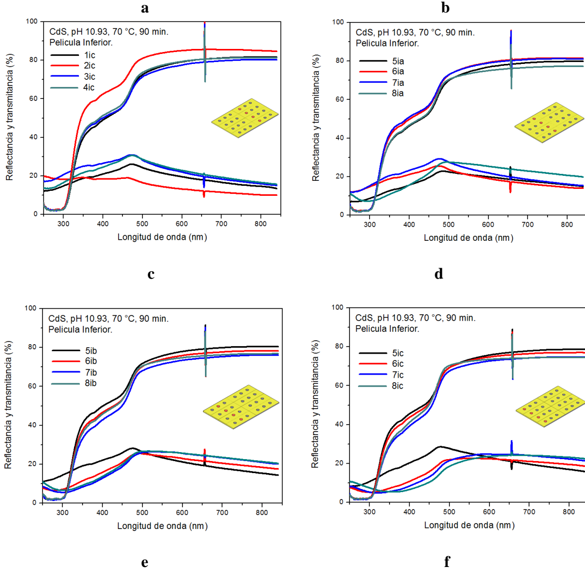
Figura 3.4. Gráficas de T&R de películas inferiores de la serie X a. 1a, 2a, 3a y 4a. b. 1b, 2b, 3b y 4b. c. 1c, 2c, 3c y 4c. d. 5a, 6a, 7a y 8a. e. 5b, 6b, 7b y 8b. f. 5c, 6c, 7c y 8c.
