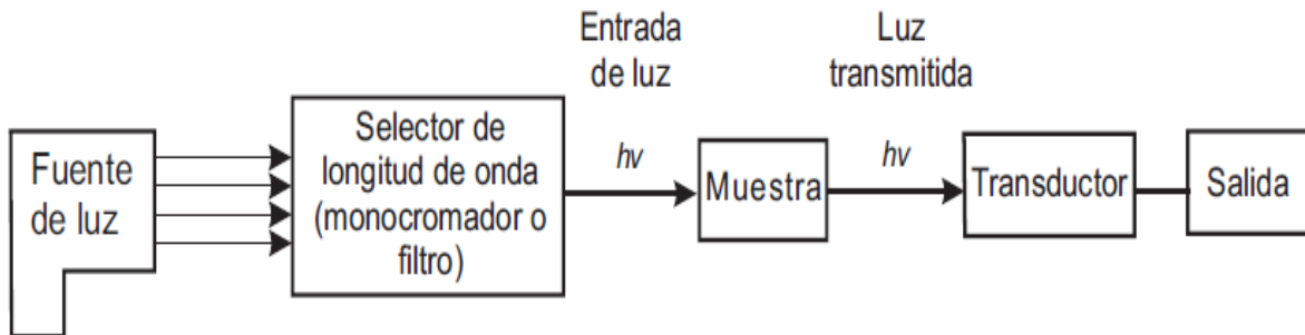
Figura 2.10. Geometría de un equipo que mide transmitancia.
