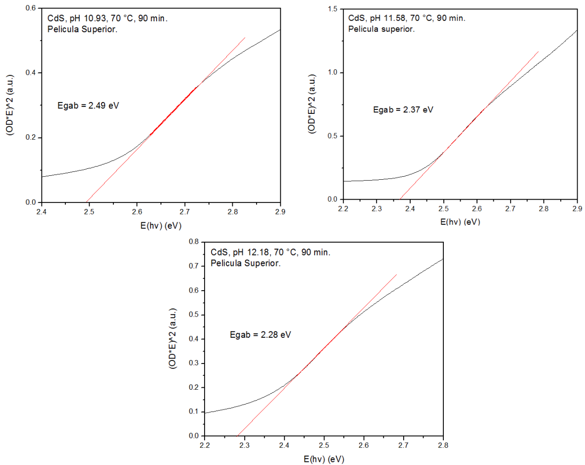
Figura 3.10. Gráfica (OD \cdot E)^2 Vs E, para obtener el E_g en la posición 3b de cada serie superior.
