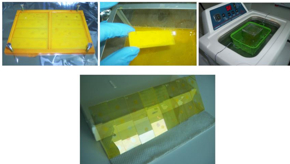
Figura 2.6. Izq. Base de naylamid con substratos después del depósito. Centro. Lavado de portaobjetos. Der. Ultrasonido. Inf. Películas de CdS después del secado con gas nitrógeno.
