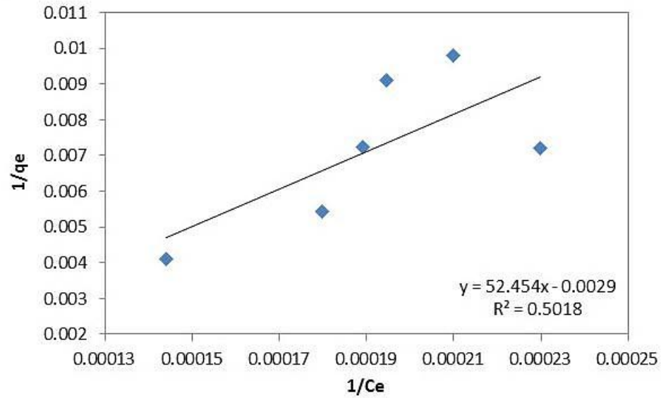
Figura 30. Isotherma de Langmuir para CA CAGR
