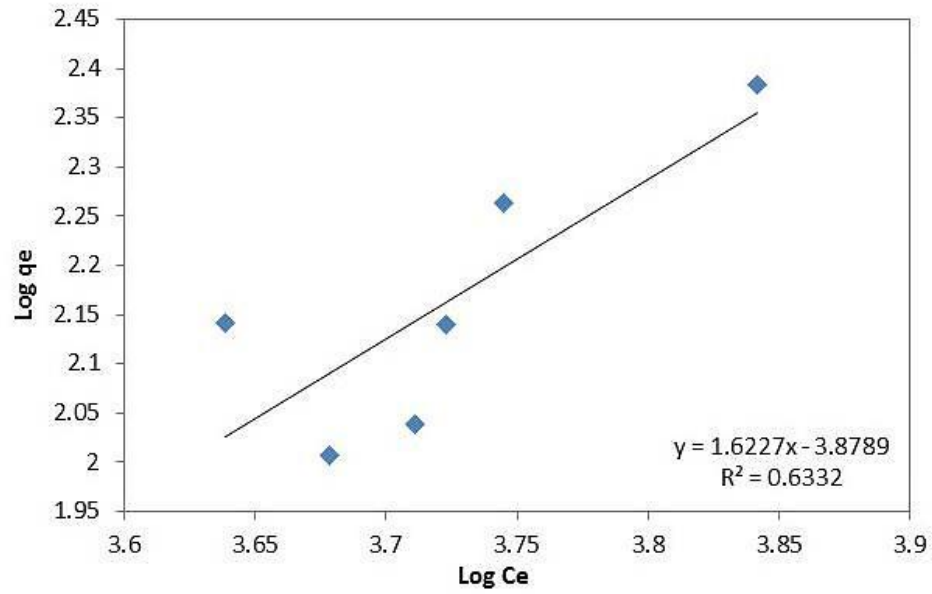
Figura 29. Isotherma de Freundlich para CA CAGR
