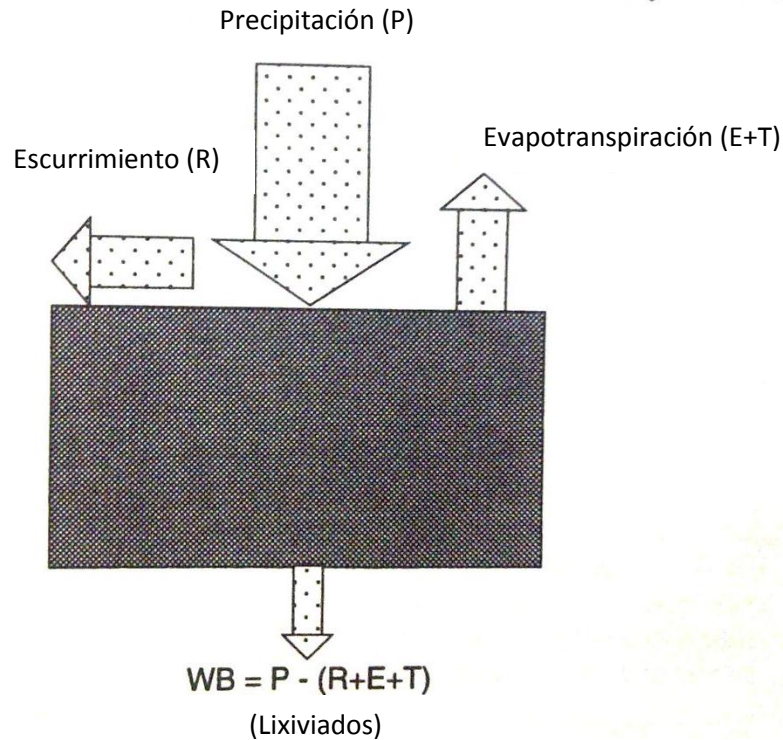
Figura 3. Balance de agua en un relleno sanitario. Fuente: Hickman, 1999.
