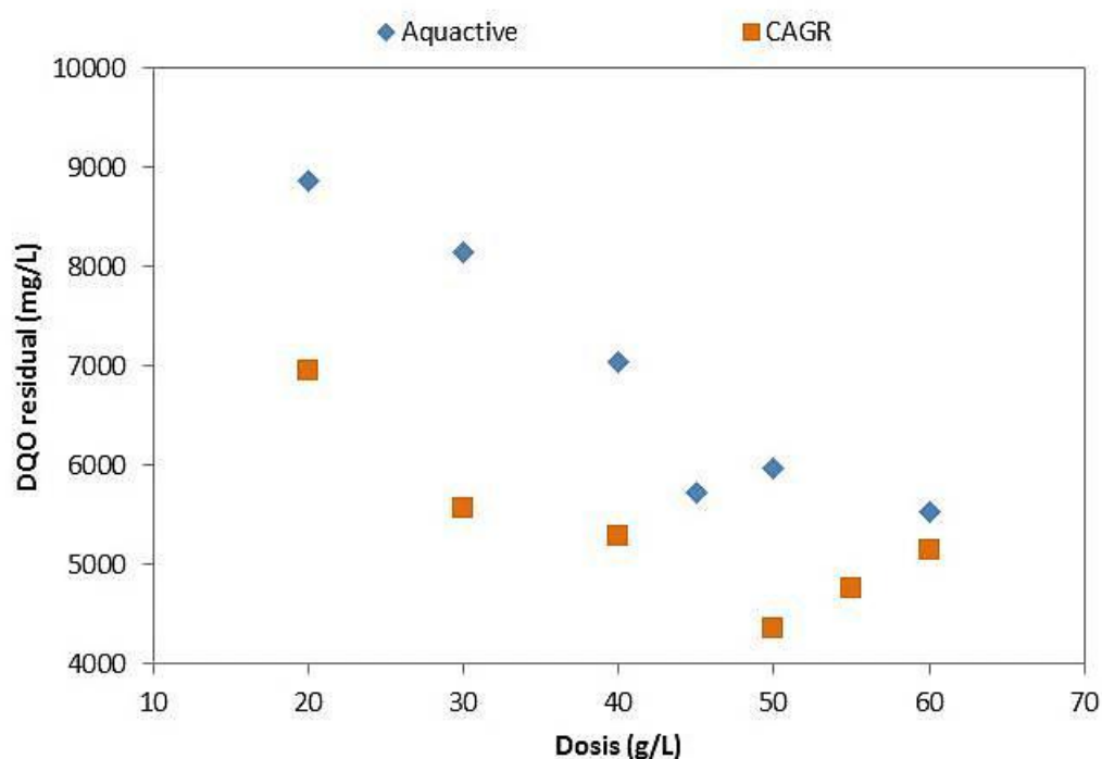
Figura 26. Efecto de CA y dosis
