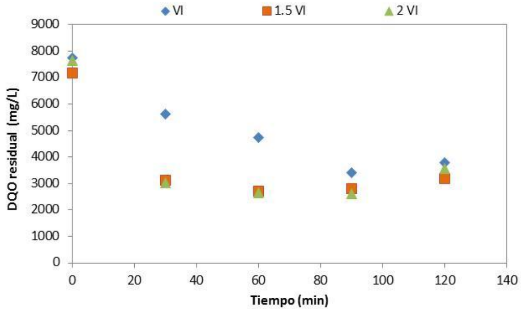
Figura 33. Efecto del incremento en las dosis de \text{H}_2\text{O}_2 y \text{Fe}^{2+} en la DQO residual a una relación molar \text{H}_2\text{O}_2/\text{Fe}^{2+} = 3
