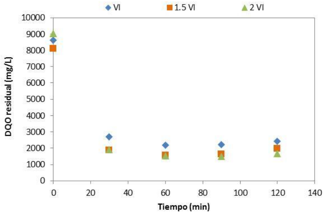
Figura 32. Efecto del incremento en las dosis de \text{H}_2\text{O}_2 y \text{Fe}^{2+} en la DQO residual a una relación molar \text{H}_2\text{O}_2/\text{Fe}^{2+} = 1.5
