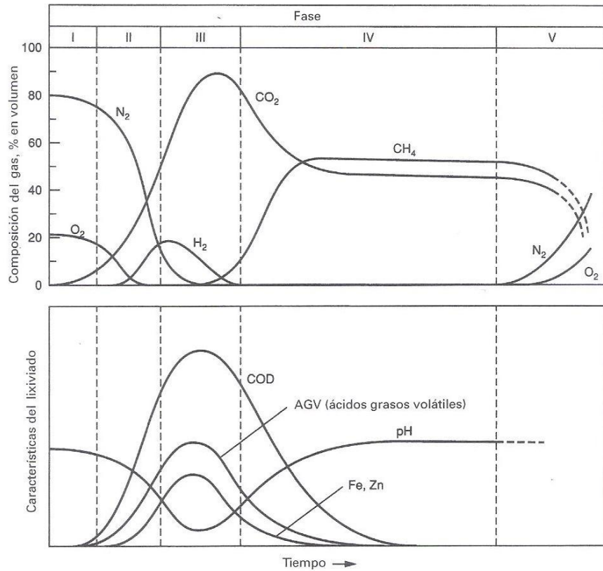
Figura 2. Fases generales en la generación de gases de vertedero (I = ajuste inicial, II = fase de transición, III = fase ácida, IV = fermentación del metano y V = fase de maduración. Fuente: Tchobanoglus et al., (1996).
