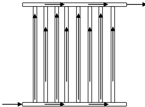
Fig. 15. Colector de cama plana.
