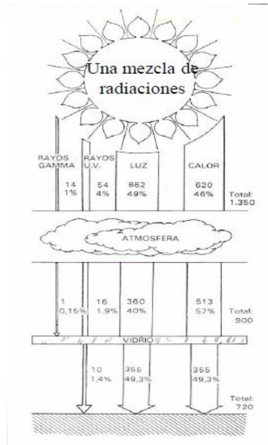
Fig. 2. Radiación Solar.
