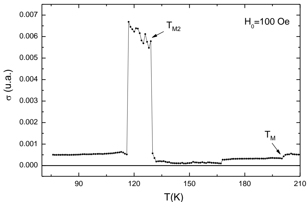
Figura 4.13. Análisis termomagnético de la Muestra Ru-1222.
