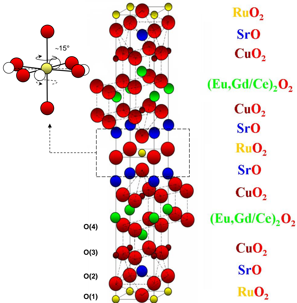
Figura 2.6: Estructura cristalina del compuesto RuSr_2(R,Ce)_2Cu_2O_{10} , donde R = Eu,Gd (Figura obtenida de Kuz',micheva, et al. , 2001 y de Lynn, et al. , 2007)
