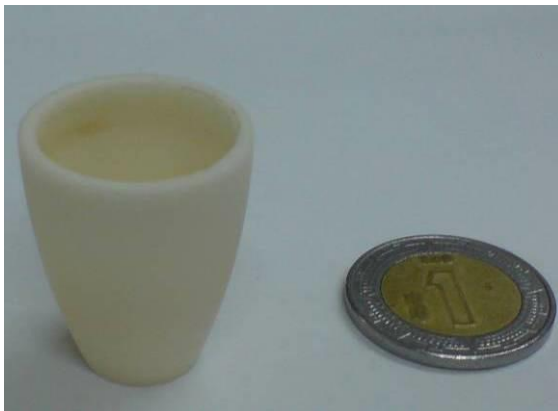
Figura 3.4. Crisol de alta alúmina utilizado durante los tratamientos térmicos intermedios.
