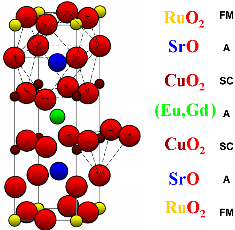
Figura 2.4: Estructura cristalina del compuesto \text{RuSr}_2\text{RCu}_2\text{O}_8 , donde R = \text{Eu, Gd} . Como se puede observar, el compuesto consiste de una secuencia alternada de capas, ordenadas a lo largo del eje c , que presentan ferromagnetismo débil (FM), que son aislantes (A) y que exhiben superconductividad (SC) (Figura obtenida de Kuz',micheva, et al. , 2001)
