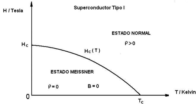
Figura 2.2. Diagrama de fases de un material superconductor Tipo I, en términos del campo magnético aplicado y la temperatura.
