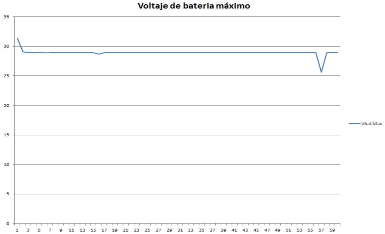
Figura 32. Gráfica: El voltaje máximo de la batería.
