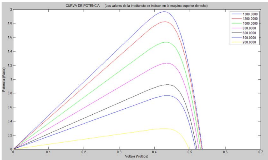
Figura 25. Octava de celdas “Curva de potencia temperatura constante 20C y irradiancia variable”
