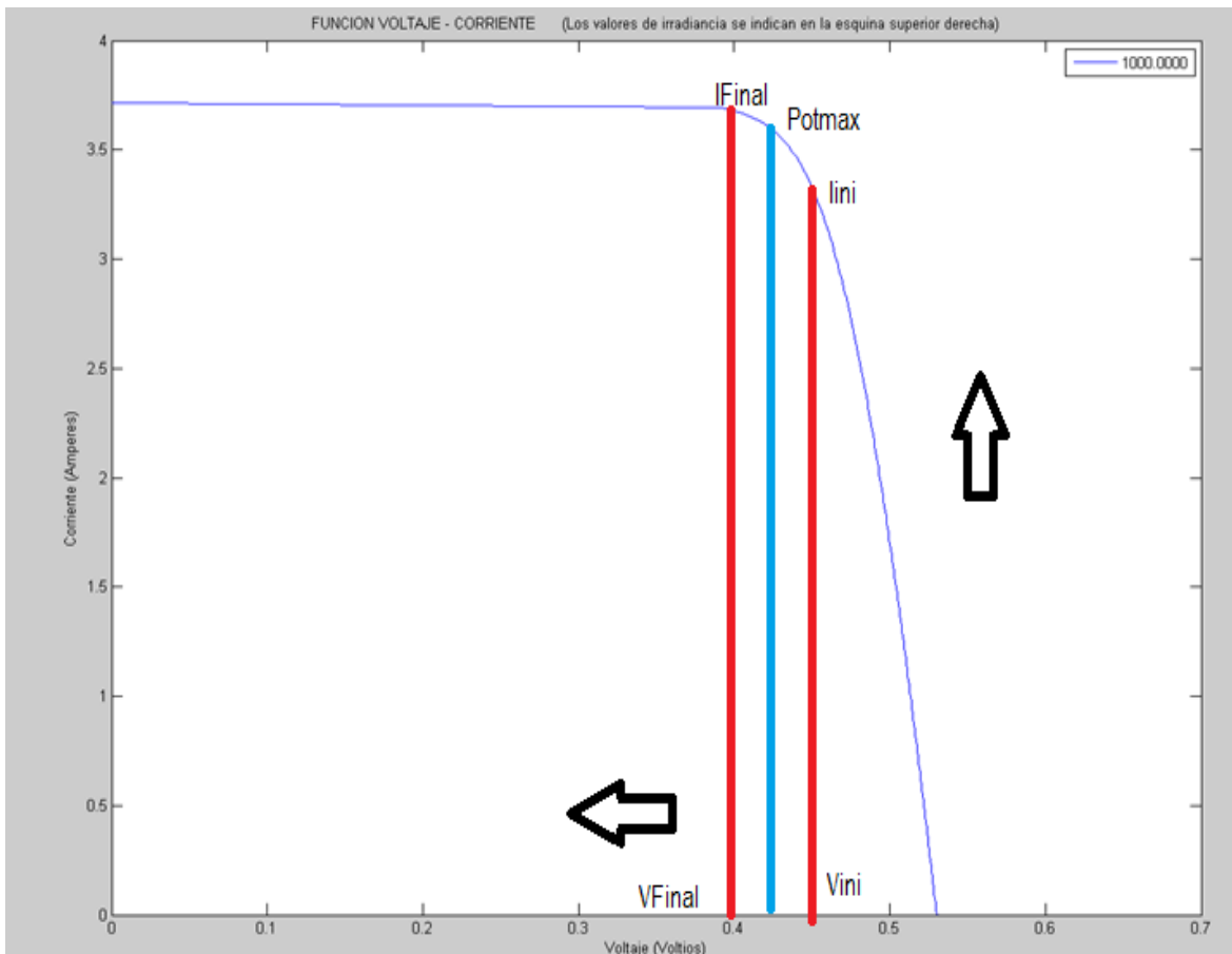
Figura 20. Potencia inicial y potencia final para aproximar a la potencia máxima.
