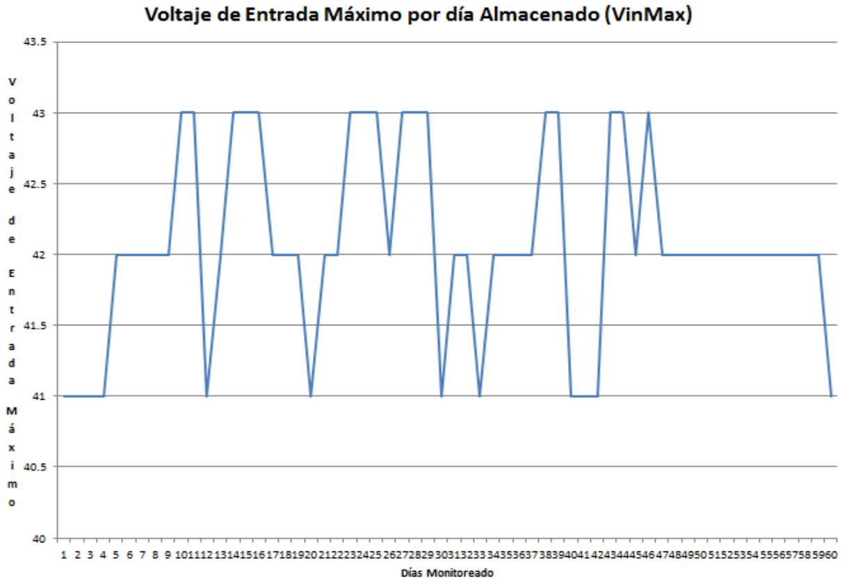
Figura 29: Gráfica: Voltaje de entrada máximo.
