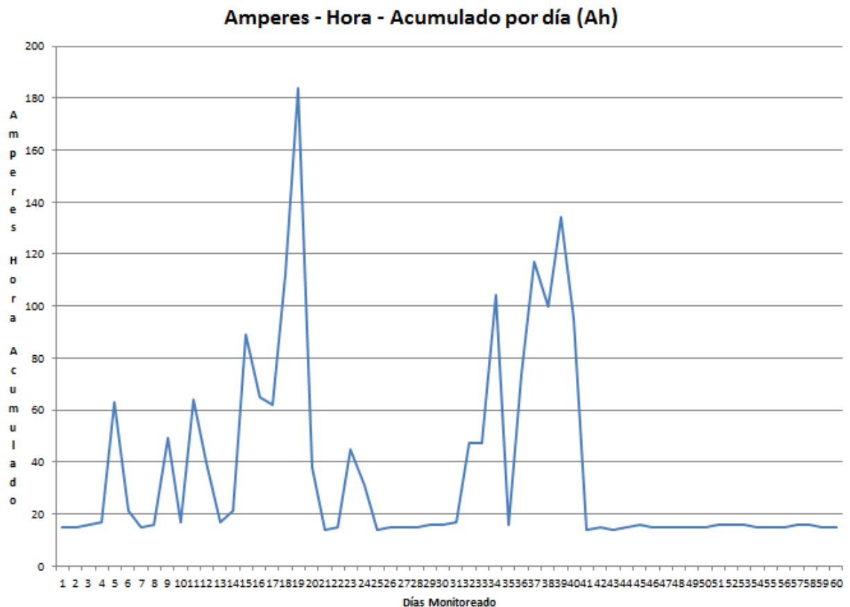
Figura 27. Gráfica: Amperes hora acumulado.
